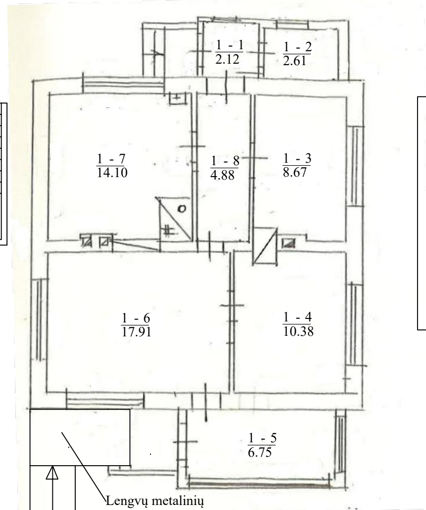
Pirmo aukšto planas
