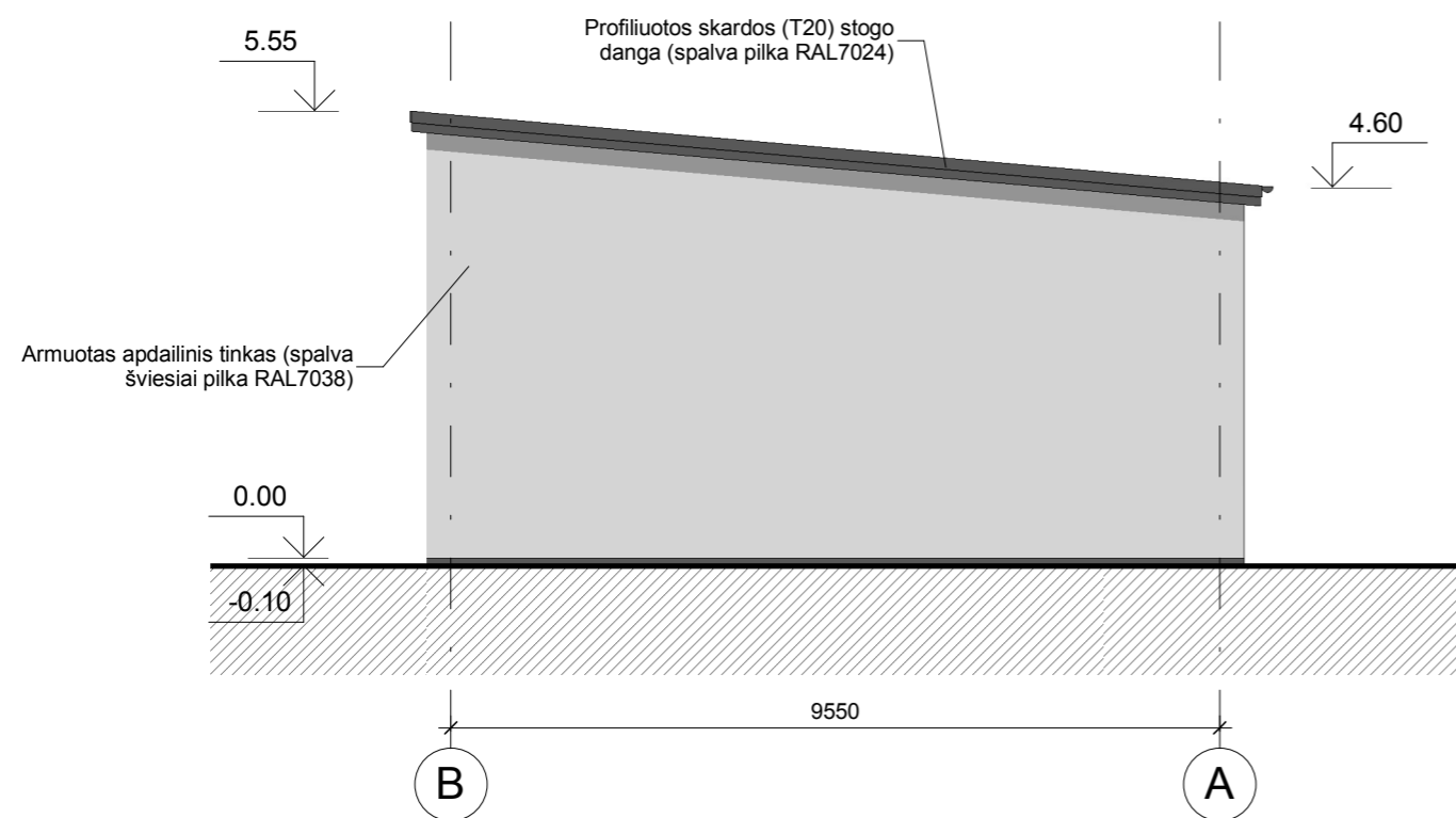
Šoninis fasadas tarp ašių B-A M 1:100
