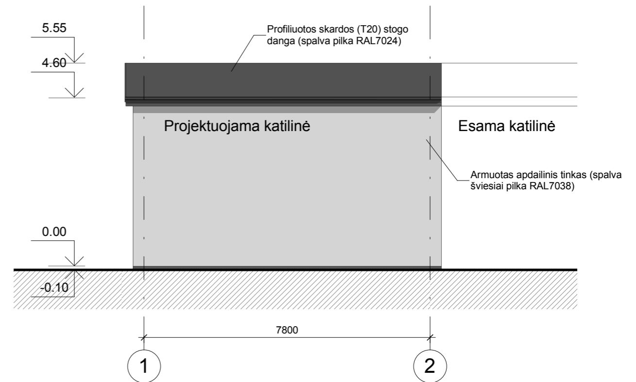
Galinis fasadas tarp ašių 1-2 M 1:100
