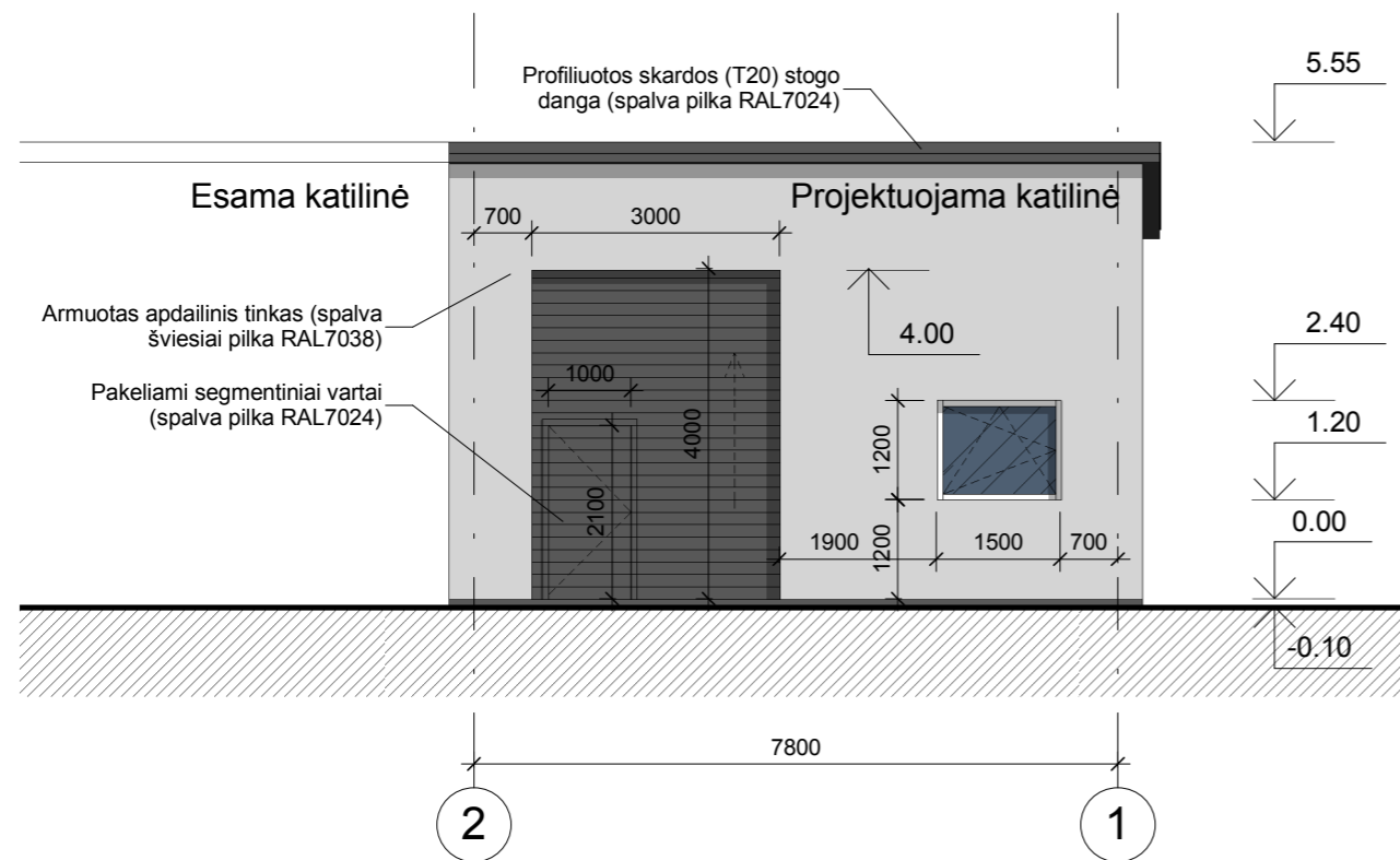
Priekinis fasadas tarp ašių 2-1 M 1:100
