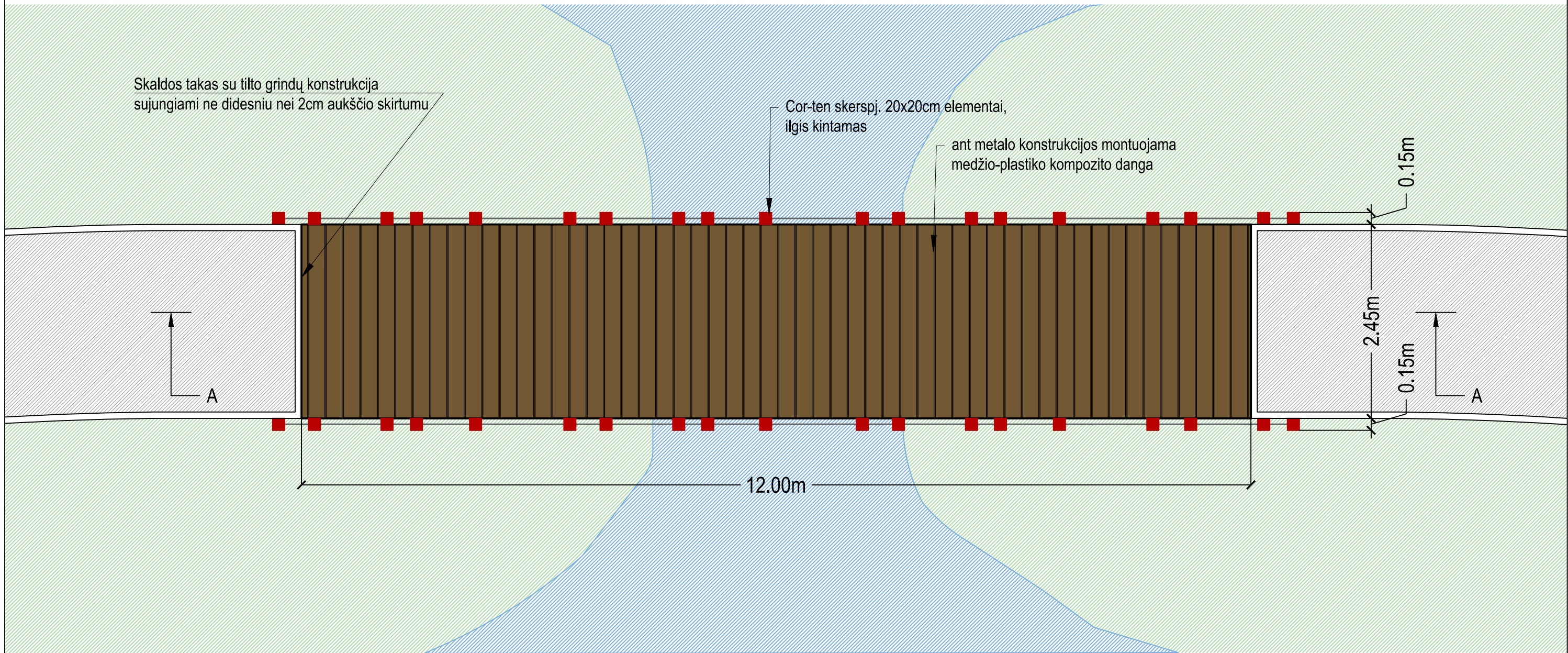
PLANAS M 1:50
