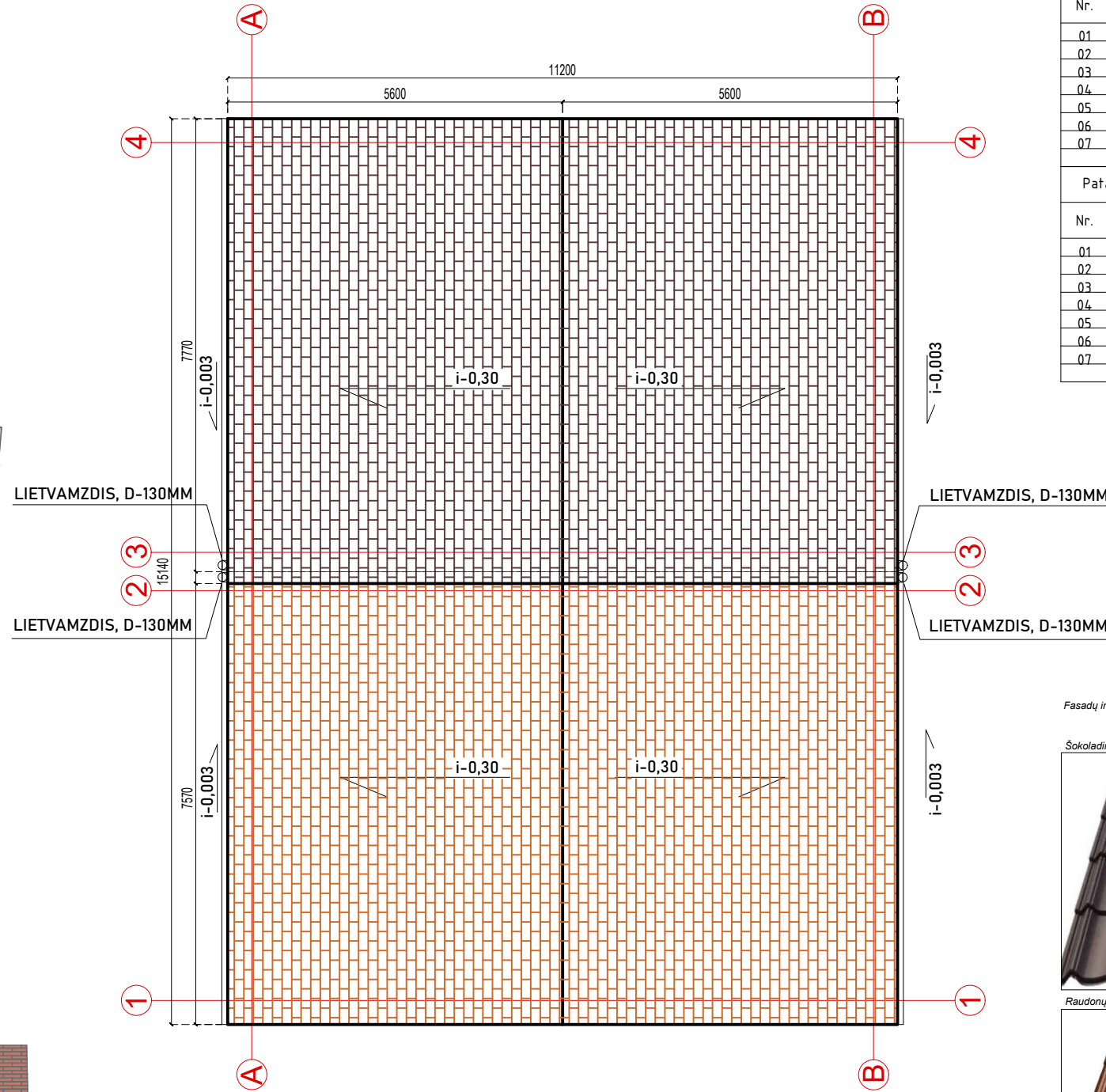
3. Stogo planas 1:100
