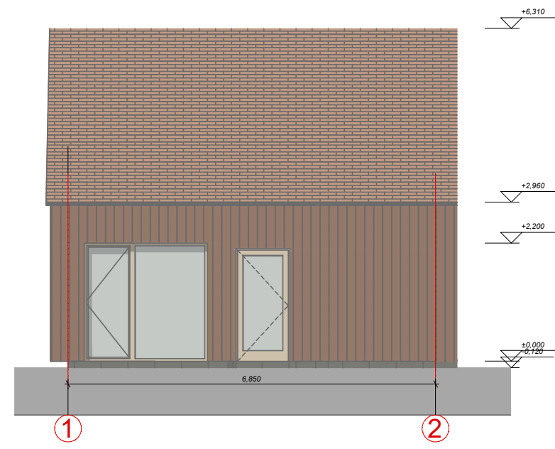
4. Rytinis fasadas 1:100
