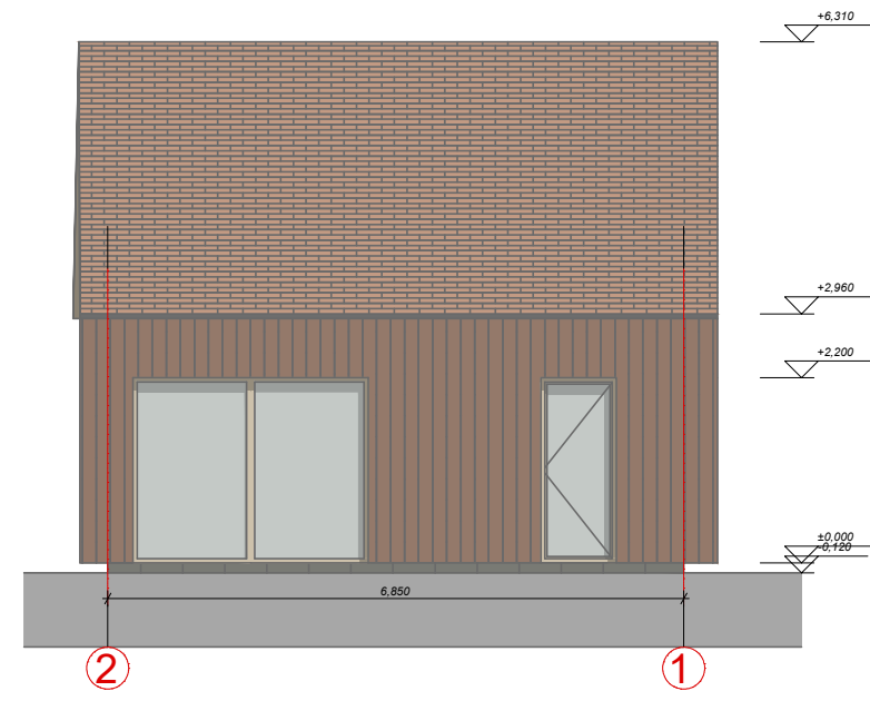
2. Vakarinis fasadas 1:100
