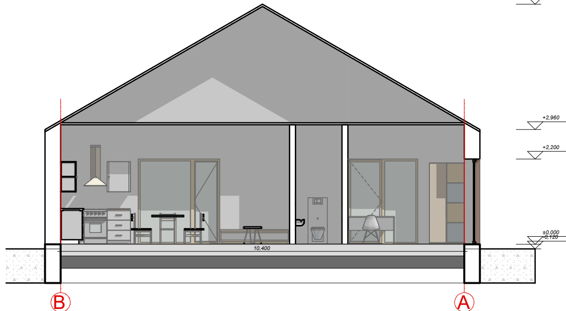
5. Pjūvis B-A 1:100
