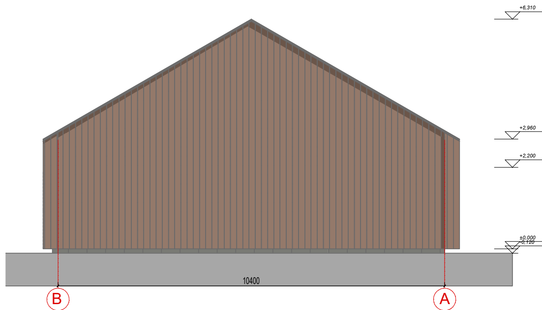
3. Šiaurinis fasadas 1:100
