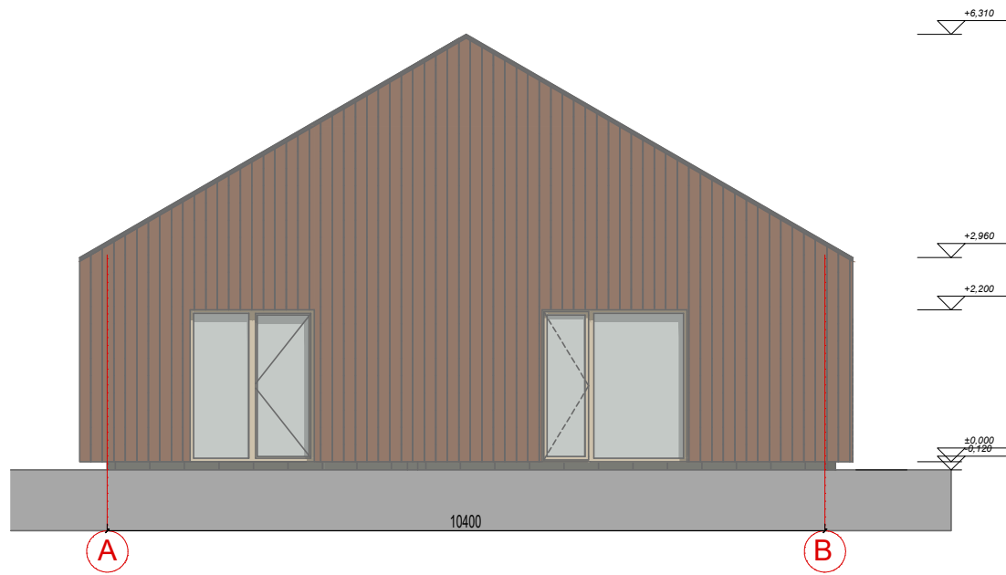
1. Pietinis fasadas 1:100
