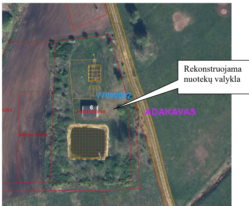
2 pav. Adakavo k. NVĮ
