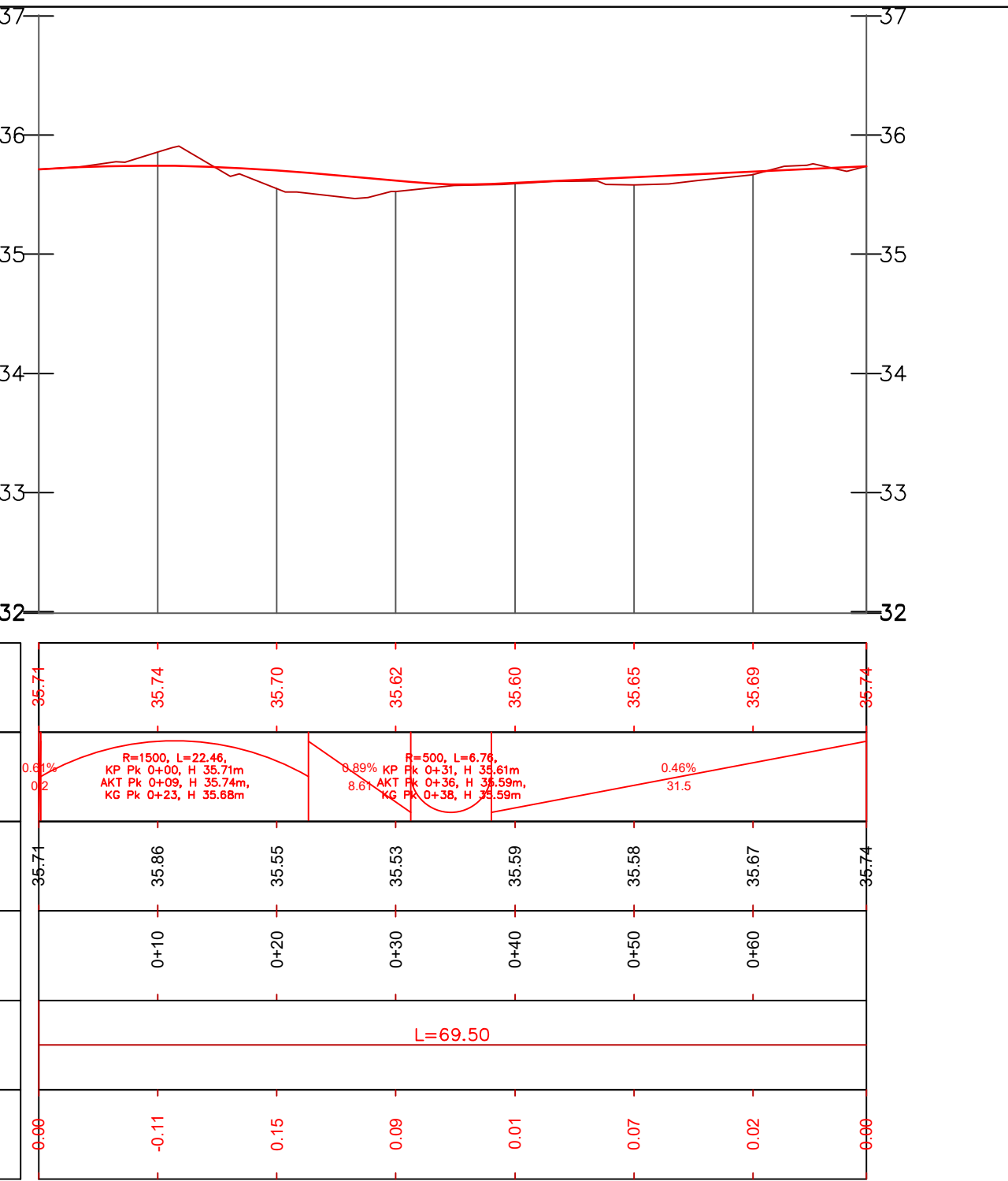
IŠILGINIS PROFILIS Mv 1:50 Mh 1:500
